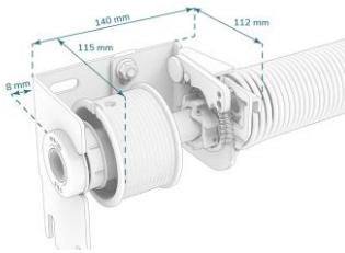
Détails Ressorts Avant :
